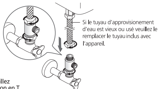
Valve de dérivation en "T"
