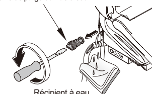
Valve de purge du filtre à eau
